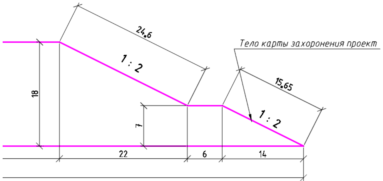
Рисунок 3.7 Схема проектного откоса карты захоронения отходов
