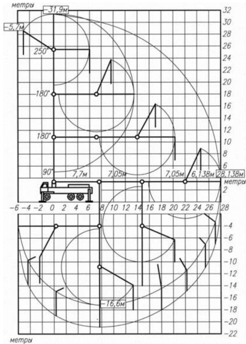
Рисунок 3.9 Характеристики автобетононасоса АБН 32
