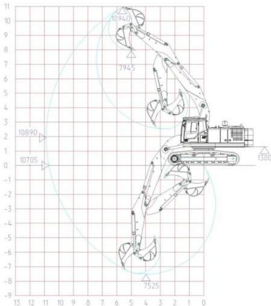
Рисунок 3.6 рабочие параметры забоя экскаватора UMG 330С
