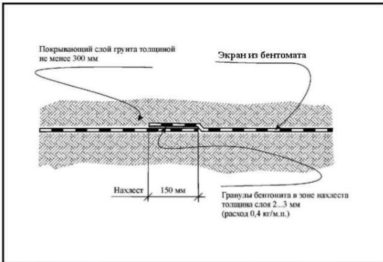
Рисунок 3.15 Герметизация зоны нахлеста
